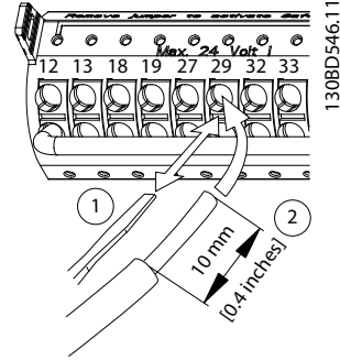
Çizim 4.10 Kontrol Tellerini Bağlama
