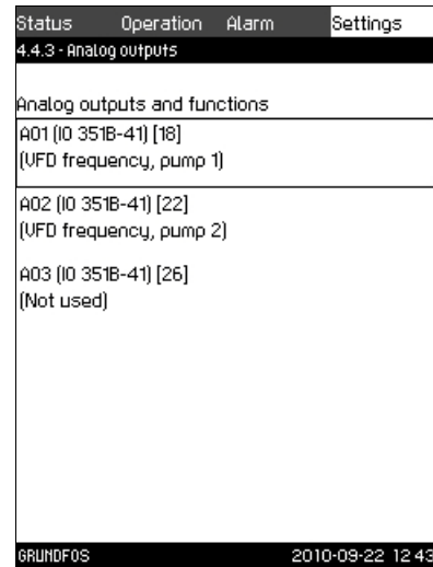
Fig. 29 Analog outputs
