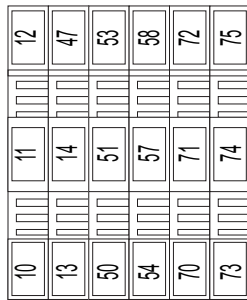
Fig. 6 Terminal block X4, CU 361
