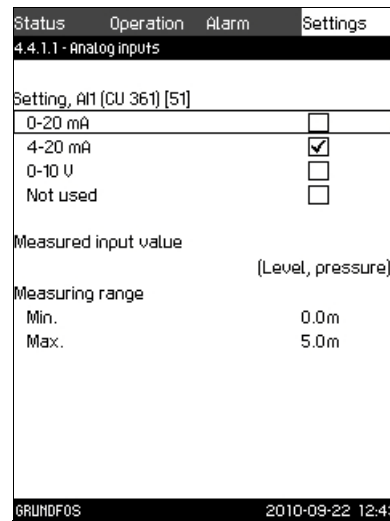
Fig. 25 Analog inputs
