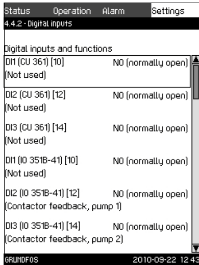
Fig. 27 Digital inputs
