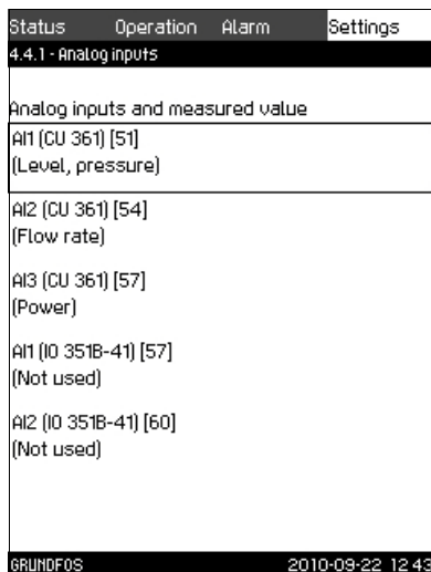
Fig. 24 Analog inputs
